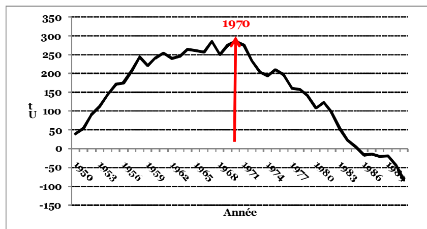
FIGURE 4 : Courbe de variation de l'indice du test de Pettit,
